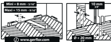
DEHNUNGSFUGENABSTAND
